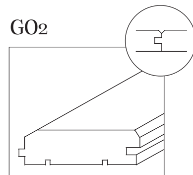
Chanfreins sur deux côtés
